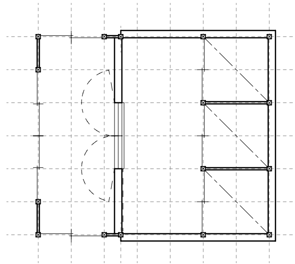
土蔵1階平面図 (S=1/100)
