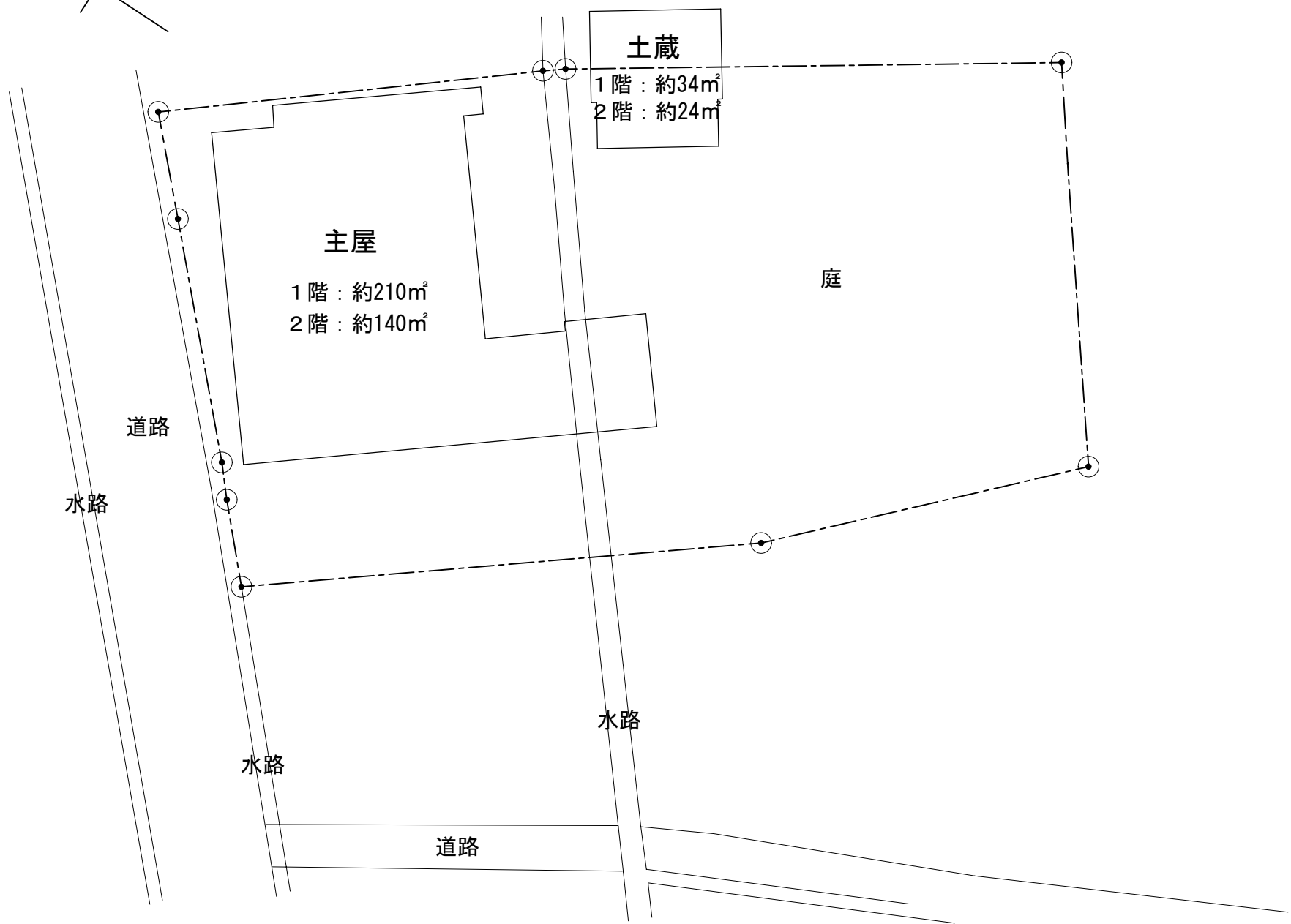
配置図 (S=1/250)
