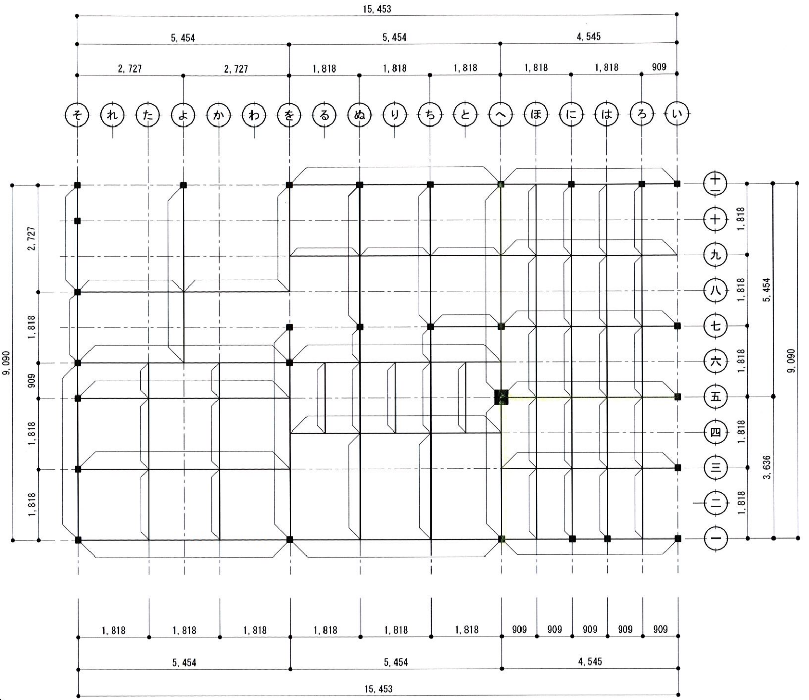
1階梁伏図 (1/100)
