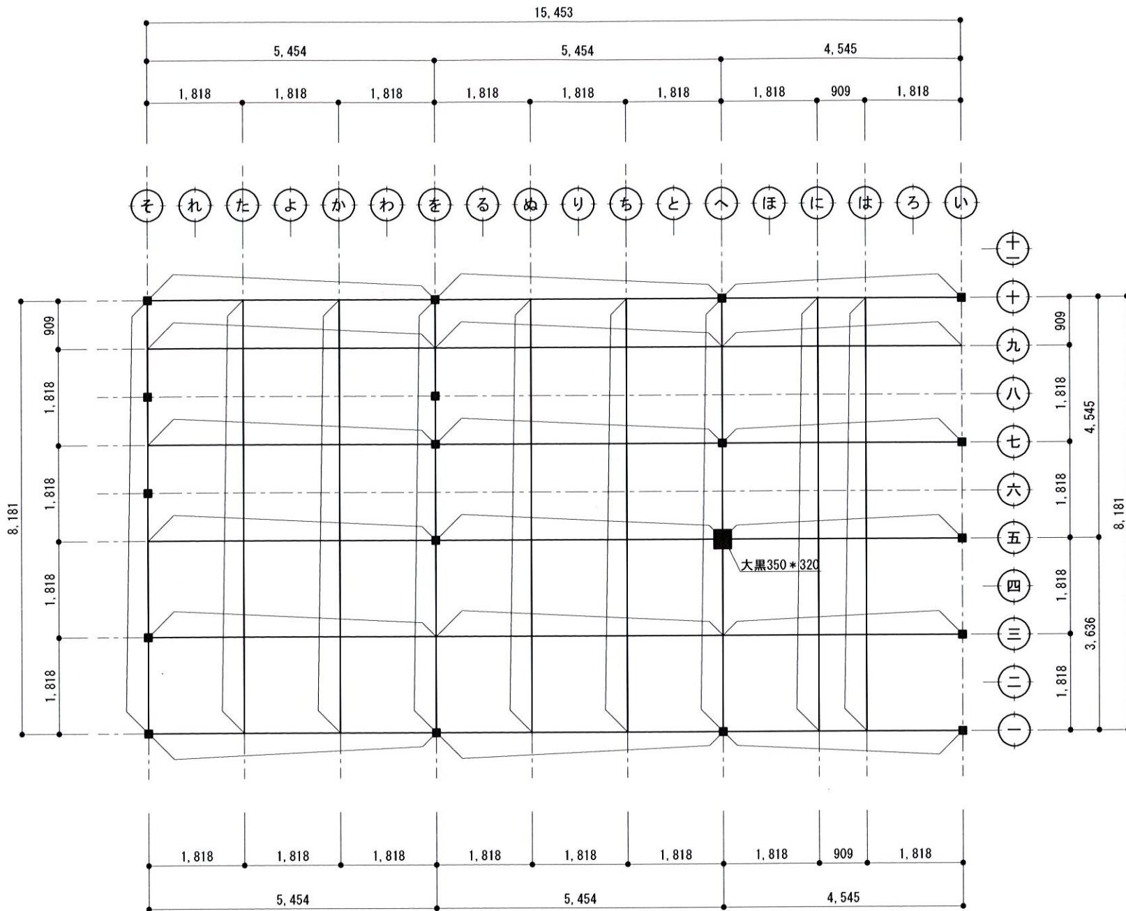
2階梁伏図 (1/100)
