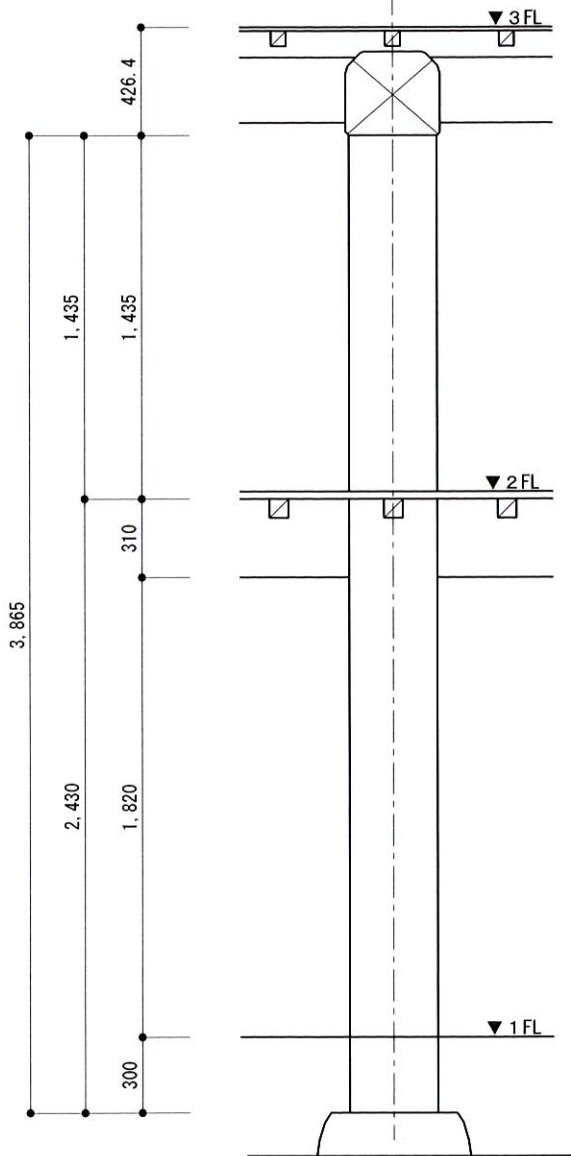
矩計図 (1/30)
