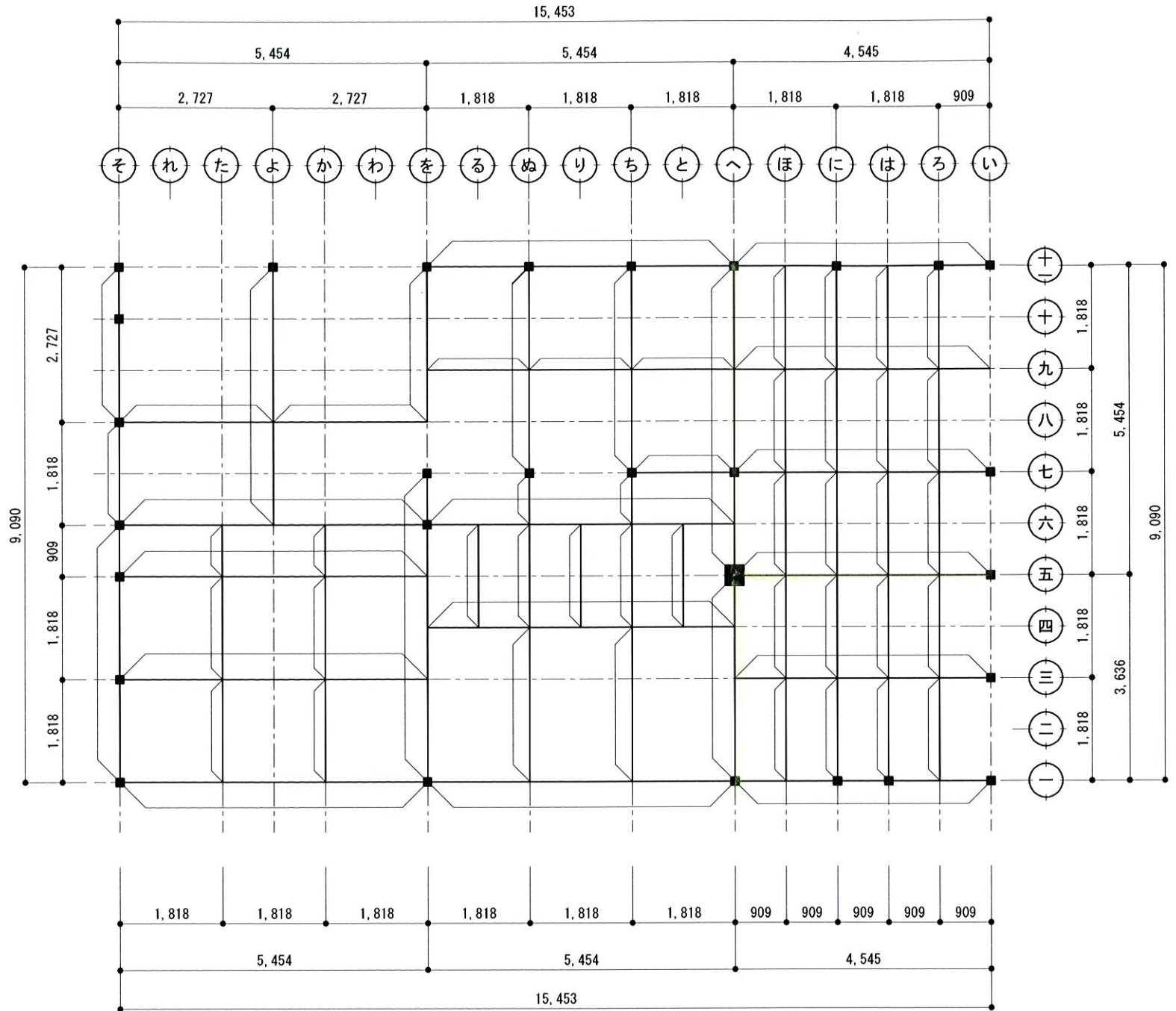
1階梁伏図 (1/100)
