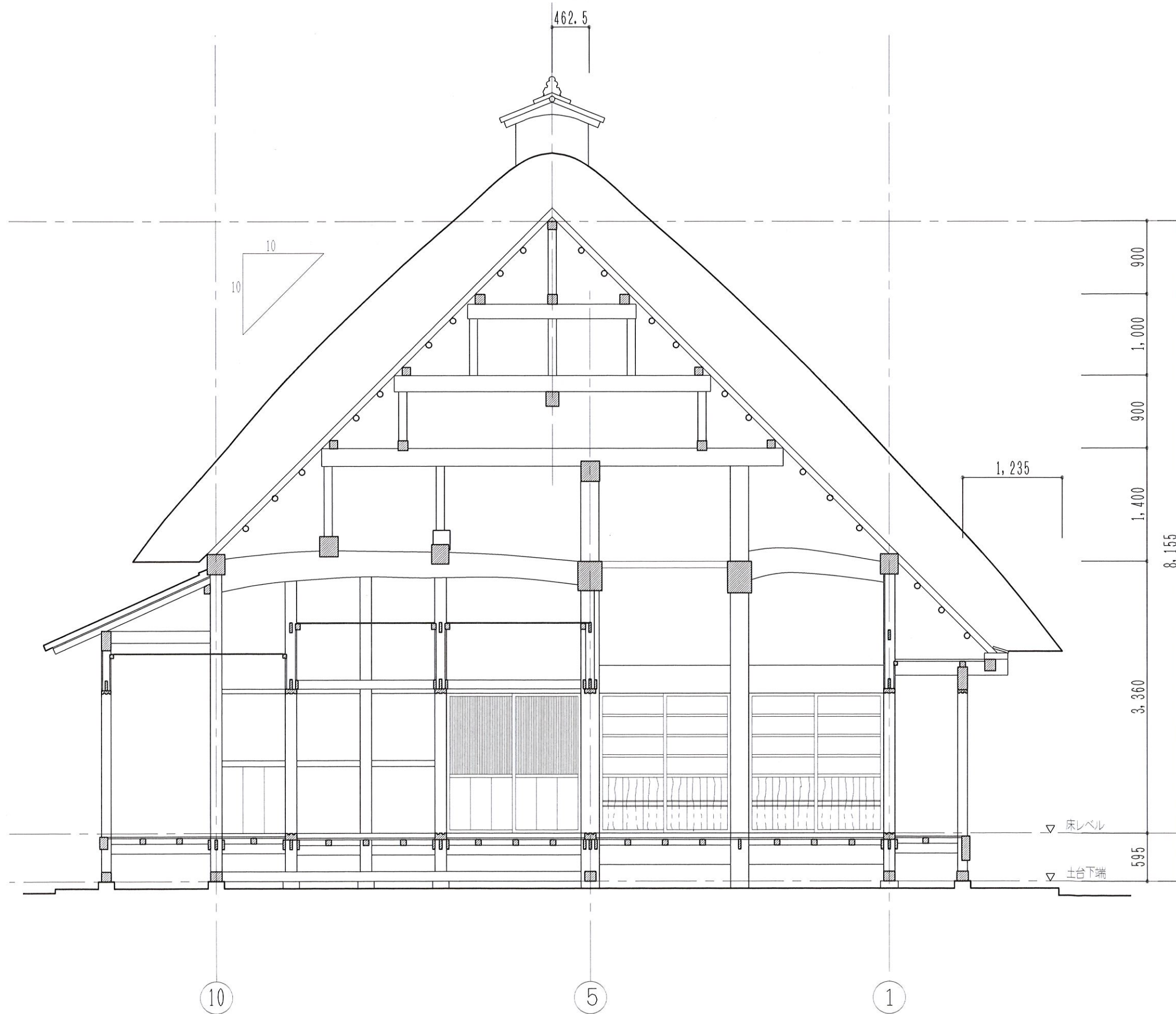
B-B' 断面図 S=1/50
