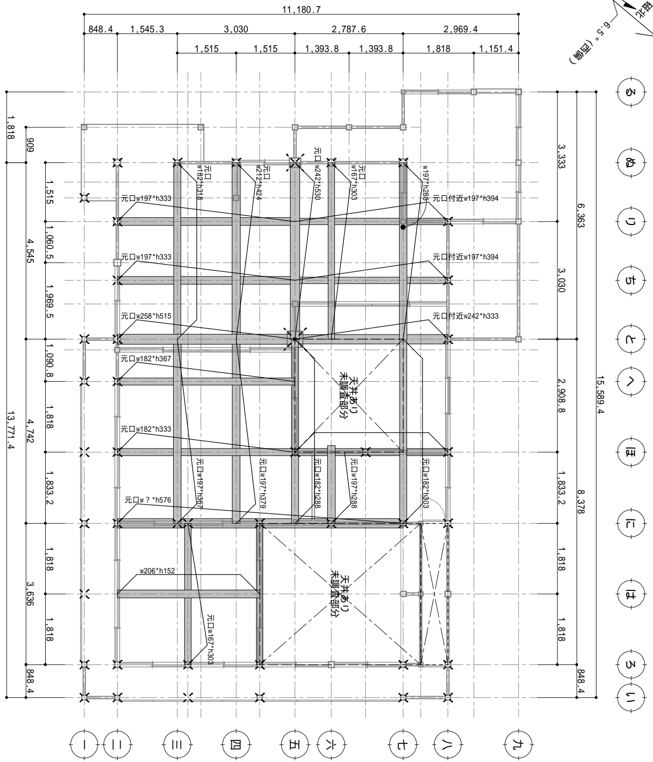
既存 下梁伏図
