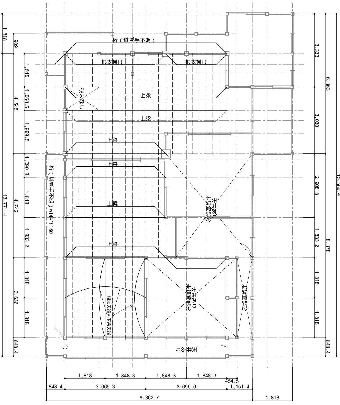
既存 上梁伏図
