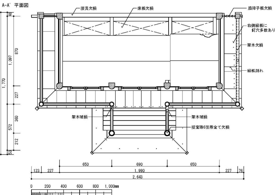
A-A' 平面図
