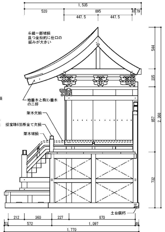
右側面図
