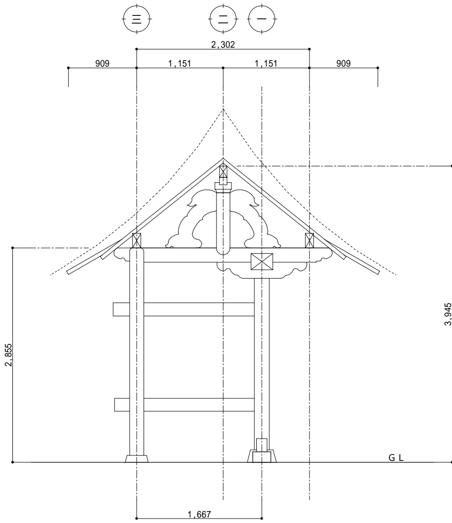
A - A ' 断面图 S=1:50
