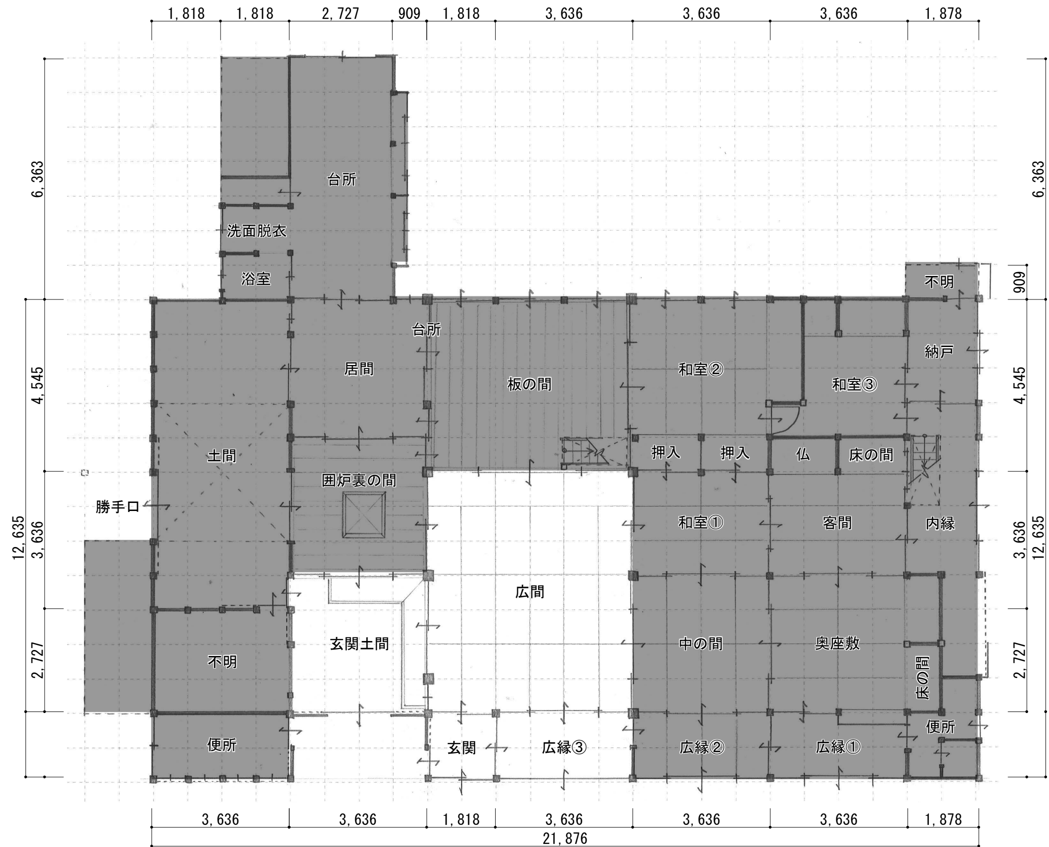
既存 平面図 S=1:100
