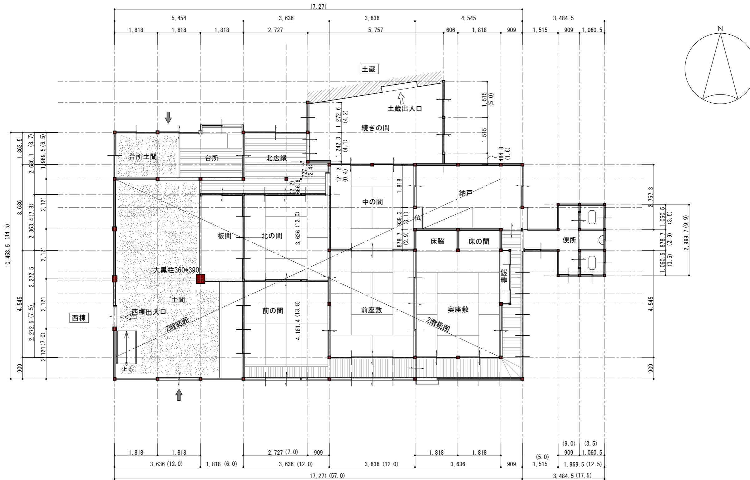
既存 1階平面図 S=1:100
