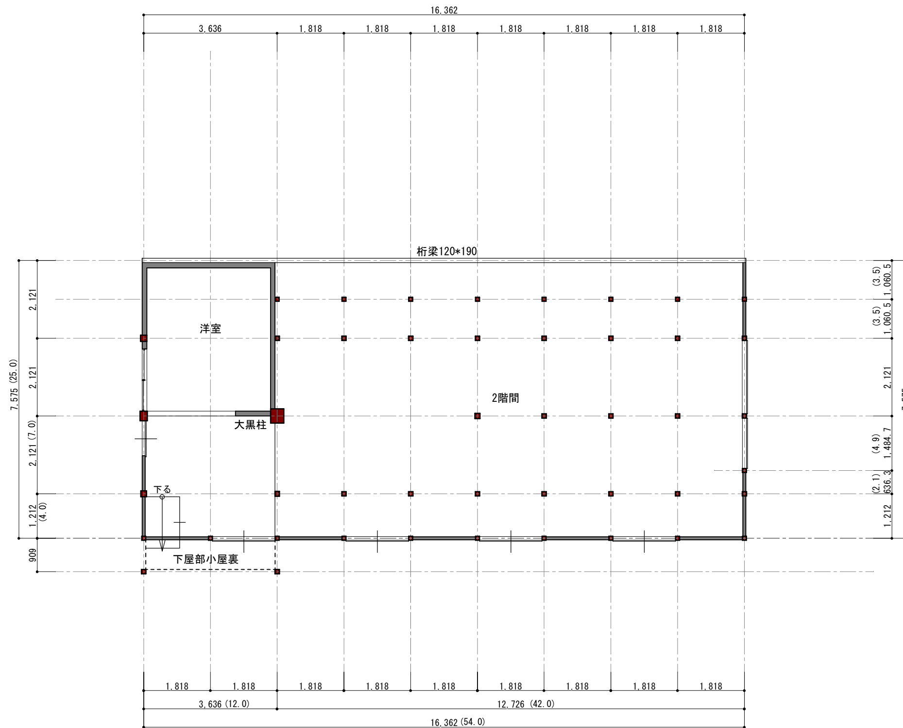
既存 2階(小屋裏) 平面図 S=1:100 柱3.5~4寸口 寸法()内数字:尺
